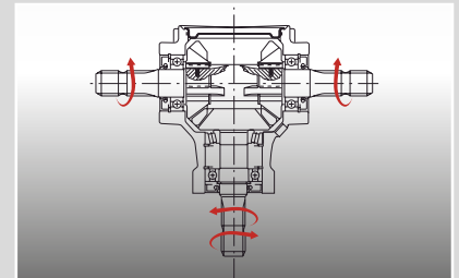
Gruppo rinvio con doppia ruota libera per trattori con guida reversibile (opzionale). Gearbox with integrated double free wheel for tractors with reversible drive (optional). Cáster de doble rueda libre para tractores de conducción reversible.
